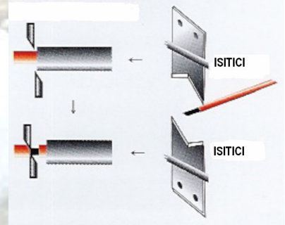
Bıçak Isıtma Ünitesi
